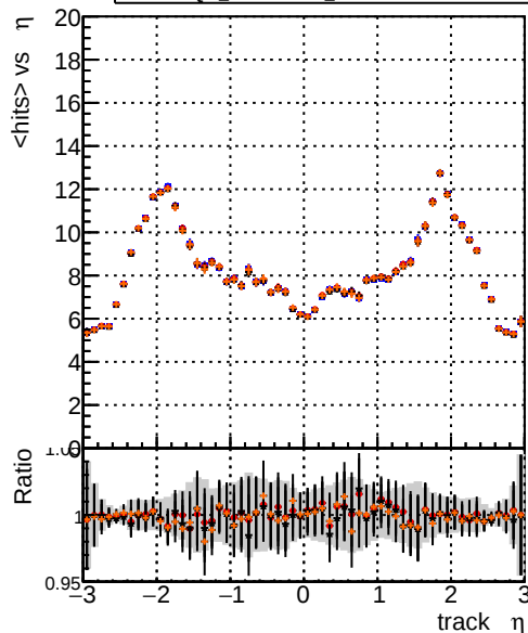
mean hits vs \eta DOM_CKFFit_1000evt DOM_CKFREFit_1000evt DOM_MkFitREFit_1000evt DOM_TESTOLHIT_1000evt
