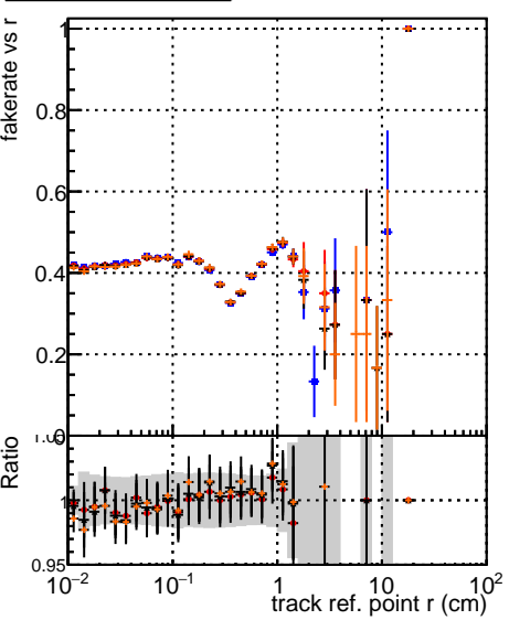
Fake rate vs —●— DQM CKFIT 1000evt —●— DQM MKEFIT 1000evt —●— DQM TESTFIT 1000evt —●— DQM OHIT 1000evt
