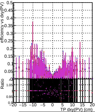
Efficiency vs Dxy(PV) Legend: DQM_CKFit-test_1000evt DQM_CKFitREFit-test_1000evt DQM_mkFitREFit-test_1000evt DQM_NANTESTCKF_1000evt DQM_NANTEST_1000evt
