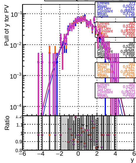
RecoPVAssoc
