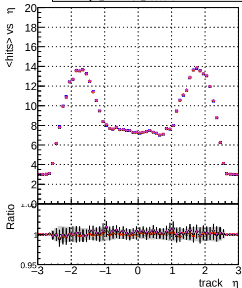
mean hits DOM CKF-test 1000evt DOM CKF-test 1000evt DOM CKF-test 1000evt DOM NANTES-CKF 1000evt DOM NANTES-CKF 1000evt
