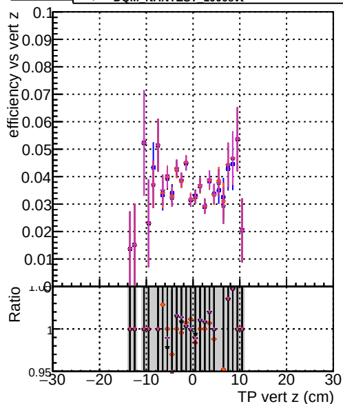
Efficiency vs vert z — DOM CKF-test 1000evt — DOM CKF-test 1000evt — DOM CKF-test 1000evt — DOM NANTESICKF 1000evt — DOM NANTES 1000evt
