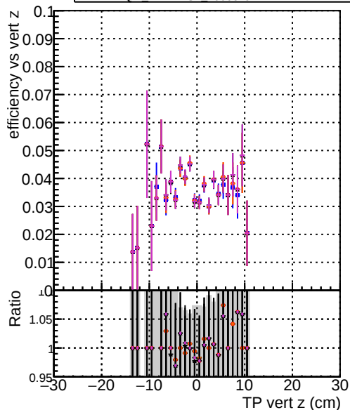
Efficiency vs vertpos — DOM CKF-test 1000evt — DOM CKFEREE-test 1000evt — DOM mkr-test 1000evt — DOM NANTESICKF 1000evt — DOM NANTEST 1000evt
