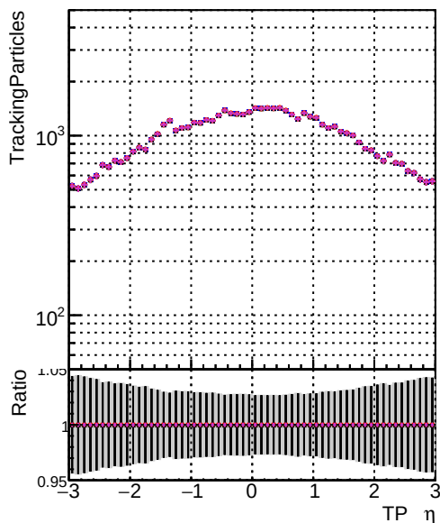
N of sin Legend DOM-mkFitREFit-test 1000evt DOM-NANTESTCKF 1000evt DOM-NANTEST 1000evt
