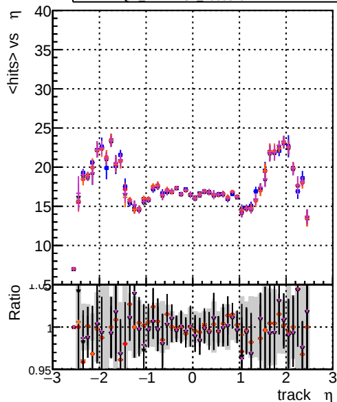
mean hits vs \eta DOM CKFERE-test 1000evt DOM CKFERE-test 1000evt DOM CKFERE-test 1000evt DOM NANTESCKF 1000evt DOM NANTES 1000evt
