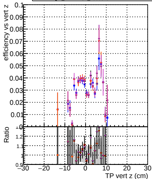
Efficiency vs vert z — DOM CKF-test 1000evt — DOM CKFERF-test 1000evt — DOM mkt-test 1000evt — DOM NANTESICKF 1000evt — DOM NANTEST 1000evt
