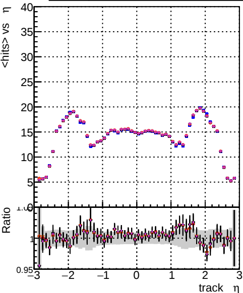
mean hits vs \eta DOM CKF-test 1000evt DOM CKF-test 1000evt DOM CKF-test 1000evt DOM NANTESCKF 1000evt DOM NANTES 1000evt
