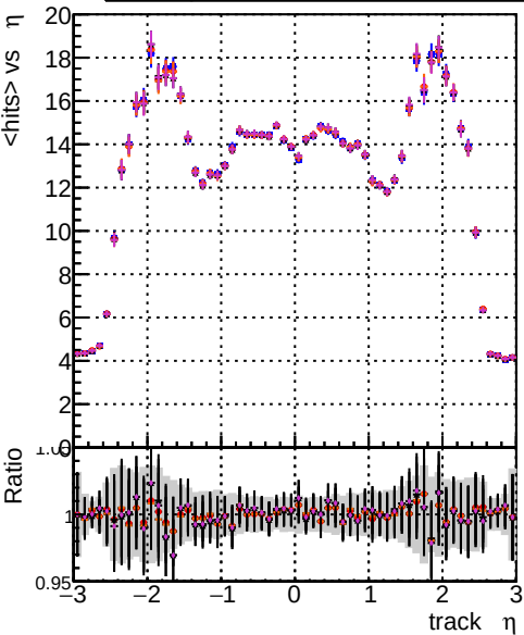
mean hit \eta DOM CKF-test 1000evt DOM CKF-test 1000evt DOM CKF-test 1000evt DOM NANTESCKF 1000evt DOM NANTES 1000evt
