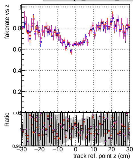
DOM CKF test 1000evt DOM CKF test 1000evt DOM CKF test 1000evt DOM NANTES 1000evt
