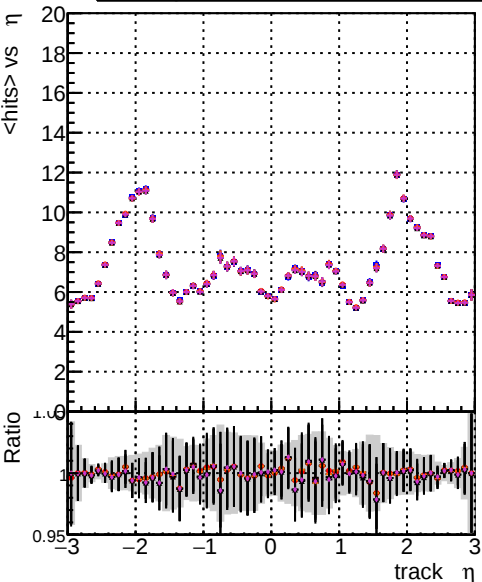
mean hits vs \eta DOM CKF-test 1000evt DOM CKF-test 1000evt DOM CKF-test 1000evt DOM CKF-test 1000evt DOM NANTESCKF 1000evt DOM NANTES 1000evt
