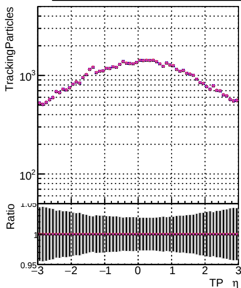
N of sin DOM CKF-test 1000evt DOM CKFit-test 1000evt DOM mkFitREFit-test 1000evt DOM NANTESTCKF 1000evt DOM NANTEST 1000evt
