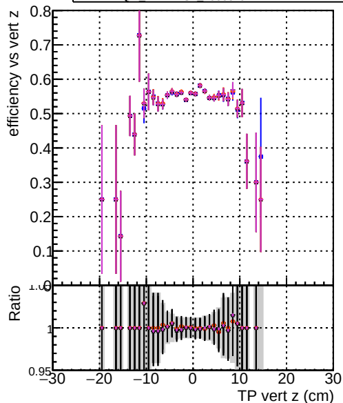
Efficiend DOM-mkFitREFit-test 1000evt DOM-NANTESTCKF 1000evt DOM-NANTEST 1000evt
