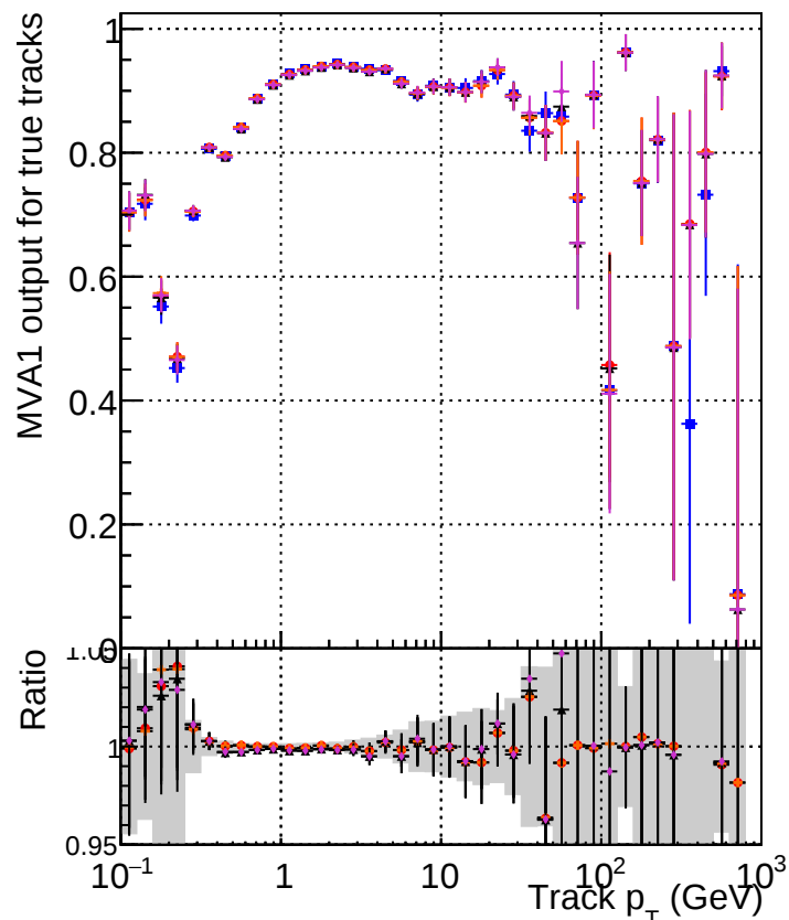
DOM_CKF-test_1000evt DOM_CKFFit-test_1000evt DOM_mkFitREFit-test_1000evt DOM_NANTESTCKF_1000evt DOM_NANTEST_1000evt
