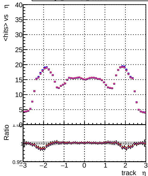
mean hits vs \eta DOM CKF-test 1000evt DOM CKF-test 1000evt DOM CKF-test 1000evt DOM NANTESICKF 1000evt DOM NANTESICKF 1000evt
