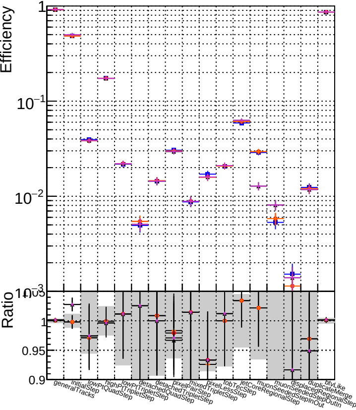
DQM_CKF-test_1000evt DQM_CKFREFit-test_1000evt DQM_mkFitREFit-test_1000evt DQM_NANTESTCKF_1000evt DQM_NANTEST_1000evt
