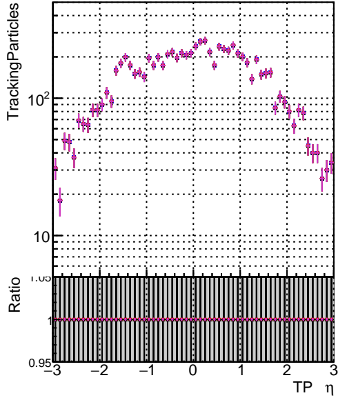
— DQM CKF-test 1000evt — DQM CKF-test 1000evt — DQM CKF-test 1000evt — DQM NANTES CKF 1000evt — DQM NANTES 1000evt
