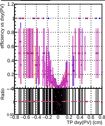
Efficiency vs Dxy(PV) Legend: DQM_CKFit-test_1000evt DQM_CKFREFit-test_1000evt DQM_mkFitREFit-test_1000evt DQM_NANTESTCKF_1000evt DQM_NANTEST_1000evt
