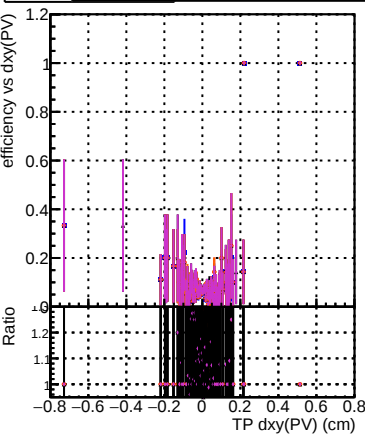
Efficiency vs Dxy(PV) DQM_CKFit-test_1000evt DQM_CKFitREFit-test_1000evt DQM_mkFitREFit-test_1000evt DQM_NANTESTCKF_1000evt DQM_NANTEST_1000evt
