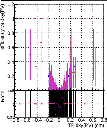
Efficiency vs Dxy(PV) Legend: DQM_CKF-test_1000evt DQM_CKFREFit-test_1000evt DQM_mkFitREFit-test_1000evt DQM_NANTESTCKF_1000evt DQM_NANTEST_1000evt
