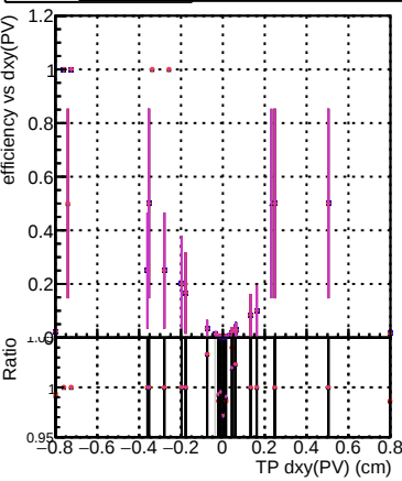
Efficiency vs Dxy(PV) DQM_CKFit-test_1000evt DQM_CKFREFit-test_1000evt DQM_mkFitREFit-test_1000evt DQM_NANTESTCKF_1000evt DQM_NANTEST_1000evt
