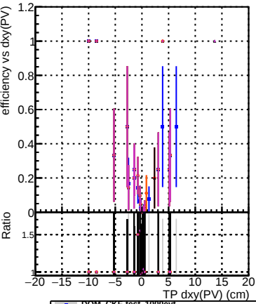
Efficiency vs Dxy(PV) DQM_CKFit-test_1000evt DQM_CKFREFit-test_1000evt DQM_mkFitREFit-test_1000evt DQM_NANTESTCKF_1000evt DQM_NANTEST_1000evt
