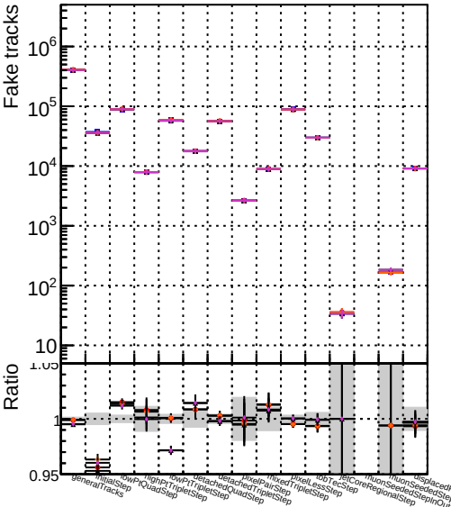
Number DOM-MIRFITREFIT-test 1000evt DOM-NANTESTCKF 1000evt DOM-NANTEST 1000evt
