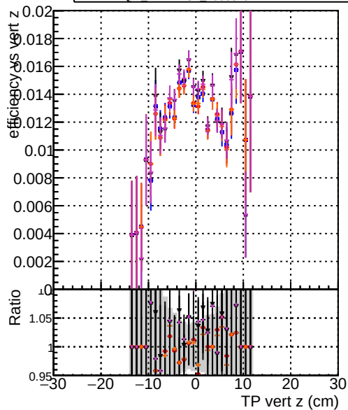
Efficiend DOM mkFitREFit-test 1000evt DOM NANTESTCKF 1000evt DOM NANTEST 1000evt
