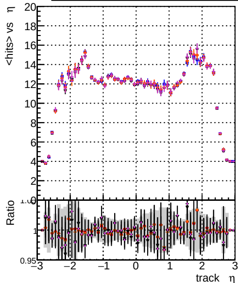
mean hits vs \eta DOM CKF-test 1000evt DOM CKF-test 1000evt DOM CKF-test 1000evt DOM NANTESCKF 1000evt DOM NANTES 1000evt
