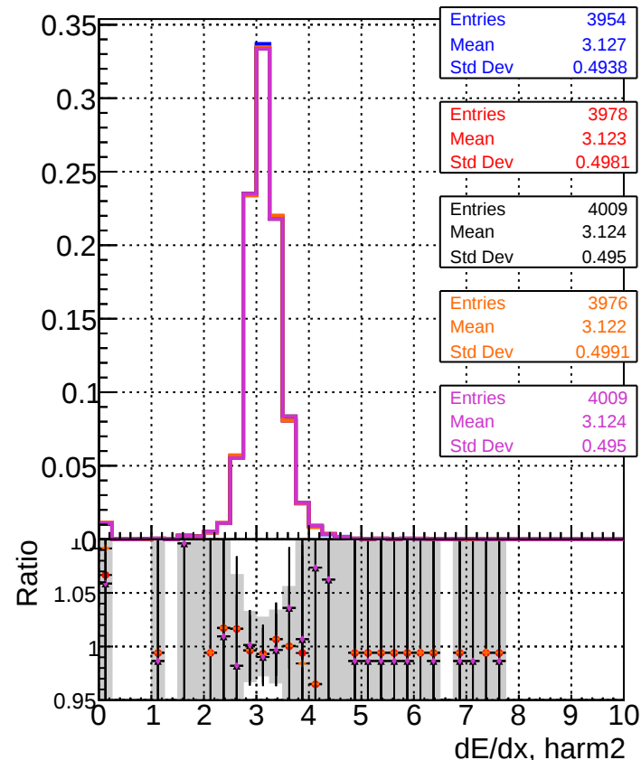
DOM_CKF-test_1000evt DOM_CKFREFit-test_1000evt DOM_mkFitREFit-test_1000evt DOM_NANTESTCKF_1000evt DOM_NANTEST_1000evt
