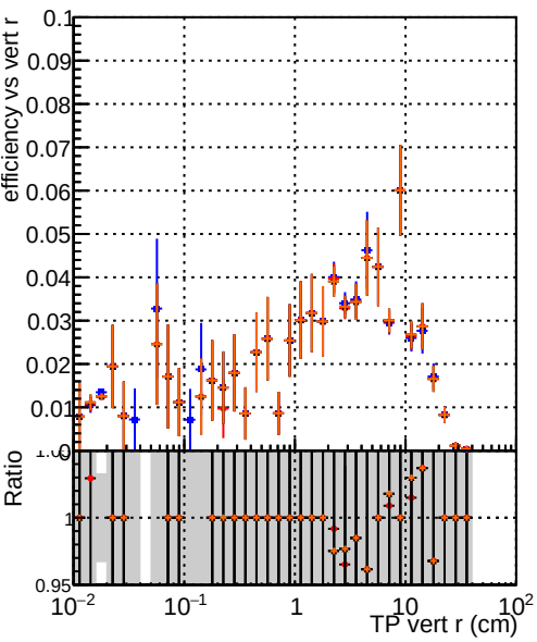
DOM_CKF-test_1000evt DOM_CKFREFit-test_1000evt DOM_mkFitREFit-test_1000evt DOM_NANTEST_1000evt
