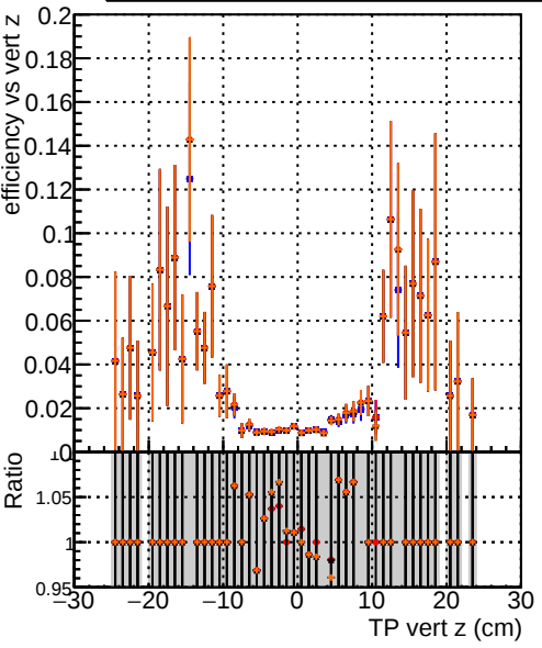
Efficiency vs vertpos DOM_CKF-test_1000evt DOM_CKFREFit-test_1000evt DOM_mkFitREFit-test_1000evt DOM_NANTEST_1000evt
