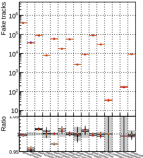
Number DQM_CKF-test_1000evt DQM_CKFit-test_1000evt DQM_mkFitREFit-test_1000evt DQM_NANTEST_1000evt
