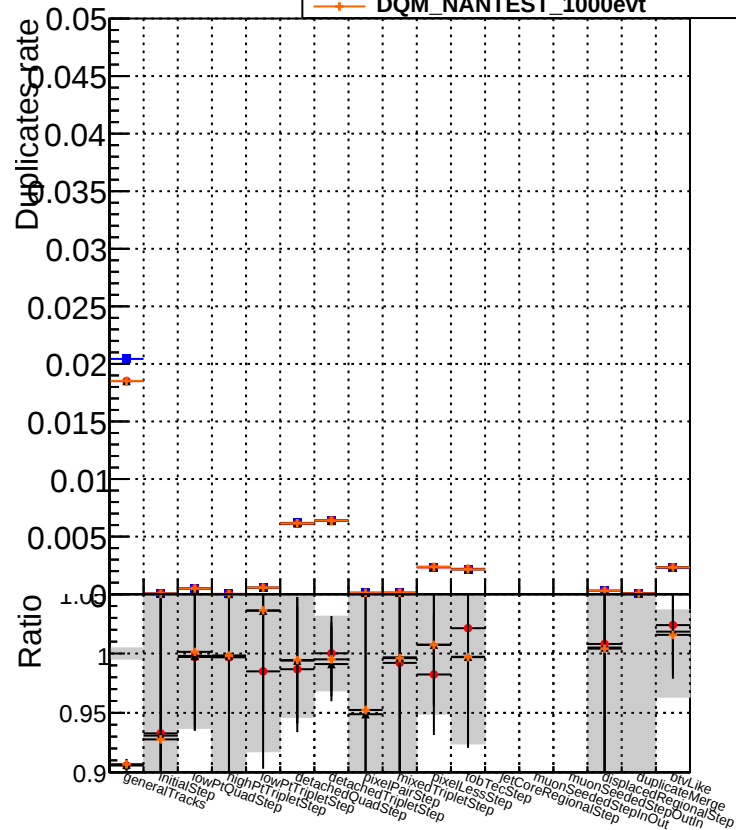
Duplicates rate vs \epsilon 0.05 —●— DQM_CKFitREFit-test_1000evt —▲— DQM_mkFitREFit-test_1000evt —+— DQM_NANTEST_1000evt
