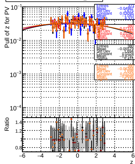
RecoPVAssoc2GenPVMatched_PullZ
