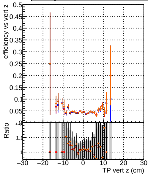
Efficiency vs vert z —•— DOM_CKF-test_1000evt —•— DOM_CKFREFit-test_1000evt —•— DOM_mkFitREFit-test_1000evt —•— DOM_NANTEST_1000evt
