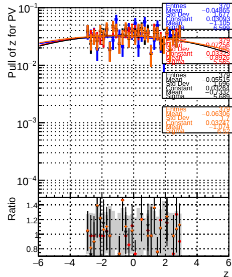
RecoPVAssoc2GenPVMatched_PulIZ
