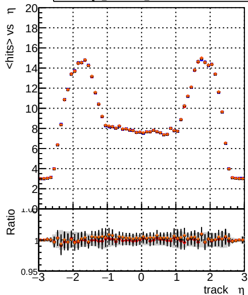
mean hits DOM_CKF-test_1000evt DOM_CKFFit-test_1000evt DOM_mkFitREFit-test_1000evt DOM_NANTEST_1000evt
