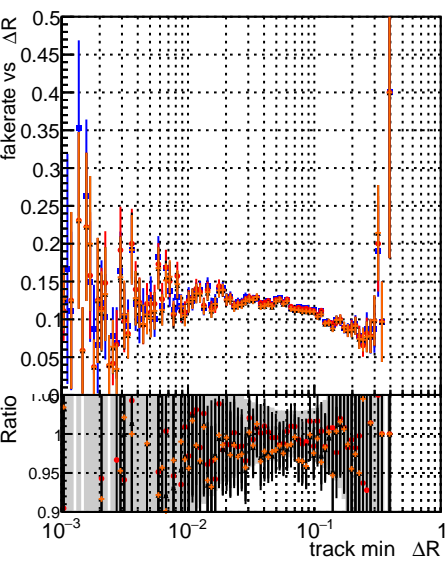
Fake rate vs \Delta R(\text{track, jet}) — DQM CKF test 1000evt — DQM CKF test 10000evt — DQM CKF test 100000evt — DQM NANTES 1000evt
