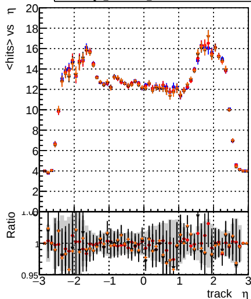
mean hits vs \eta DOM_CKF-test_1000evt DOM_CKFFit-test_1000evt DOM_mkFitREFit-test_1000evt DOM_NANTEST_1000evt
