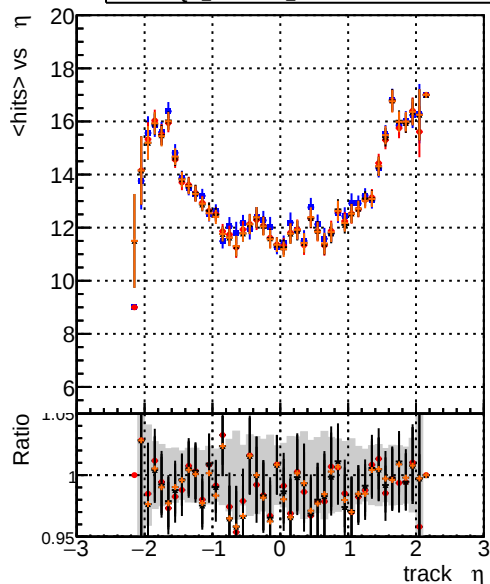
DOM_CKF-test_1000evt DOM_CKFFit-test_1000evt DOM_mkFitREFit-test_1000evt DOM_NANTEST_1000evt
