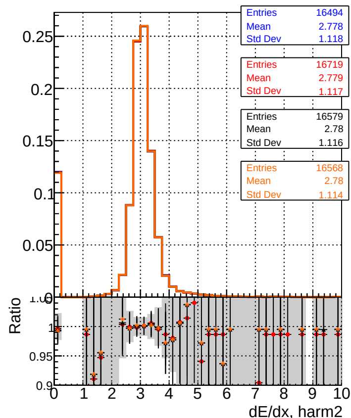
dE/dx estimator 1
