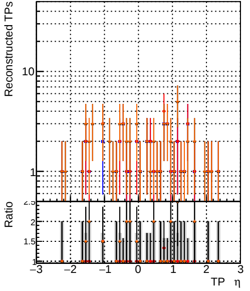
—•— DOM_CKF-test_1000evt —•— DOM_CKFFit-test_1000evt —•— DOM_mkFitREFit-test_1000evt —•— DOM_NANTEST_1000evt
