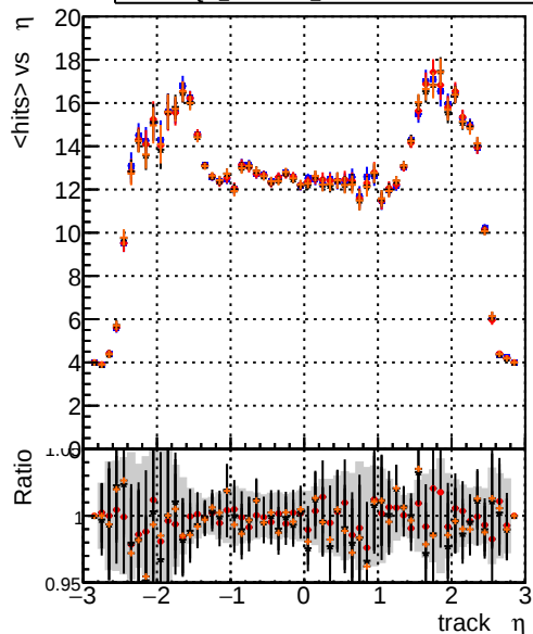
mean hits vs \eta DOM_CKF-test_1000evt DOM_CKFREFit-test_1000evt DOM_mkFitREFit-test_1000evt DOM_NANTEST_1000evt
