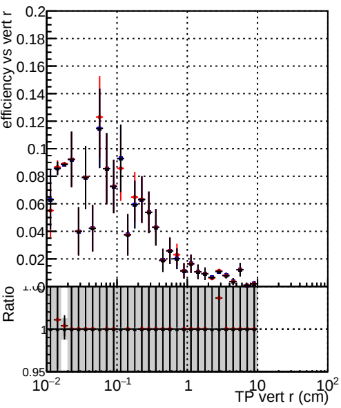
Efficiency vs TP vert r (cm) Legend: DQM_CKFFit_1000evt DQM_CKFREFit_1000evt DQM_NOTESTCKF_1000evt
