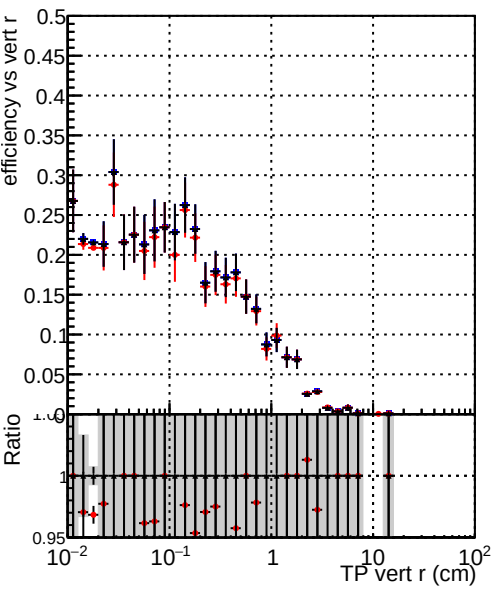
Efficiency vs TP vert r (cm) Legend: DQM_CKFFit_1000evt (blue circles) DQM_CKFREFit_1000evt (red circles) DQM_NOTESTCKF_1000evt (black circles)
