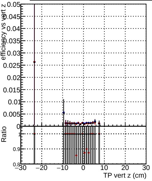
Efficiency vs vert z Legend: DQM_CKFFit_1000evt DQM_CKFREFit_1000evt DQM_NOTESTCKF_1000evt
