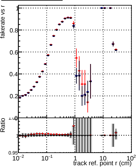
Fake rate vs vertpos DOM CKFFit 1000evt DOM CKFREFit 1000evt DOM NOTESTCKF 1000evt
