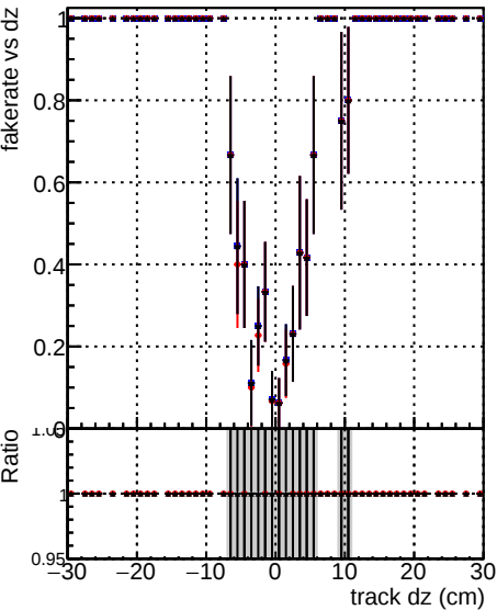
Fake rate vs dz DOM CKEEF 1000evt DOM CKEEF 1000evt DOM NOTESTCKP 1000evt
