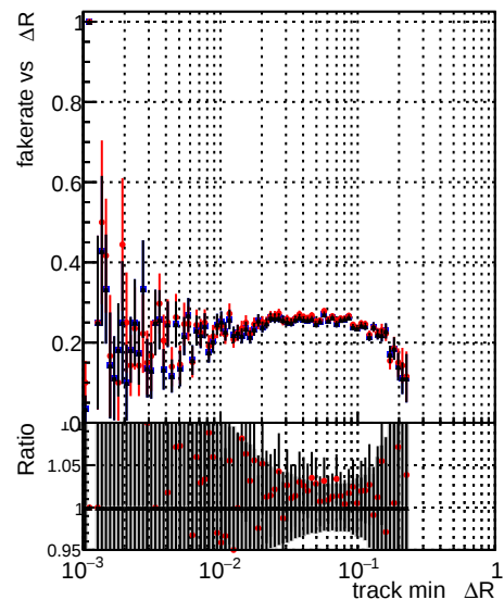
— DOM CKFFit 1000evt — DOM CKFREFit 1000evt — DOM NOTESTCKF 1000evt
