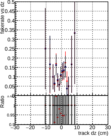
Fake rate vs dz Legend: DOM CKEEL 1000evt DOM CKEEL 1000evt DOM NOTESTCKP 1000evt
