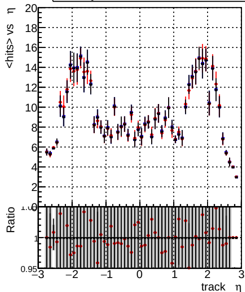
mean hit \eta — DQM_CKFFit_1000evt — DQM_CKFREFit_1000evt — DQM_NOTESTCKF_1000evt
